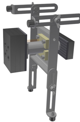
9533079007 DISPOSITIVO COLLAUDO CILINDRI MANIGLIONI RESTRAINT ACTUATORS TEST DEVICE
